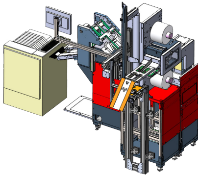
Autoslip - Top Apply
